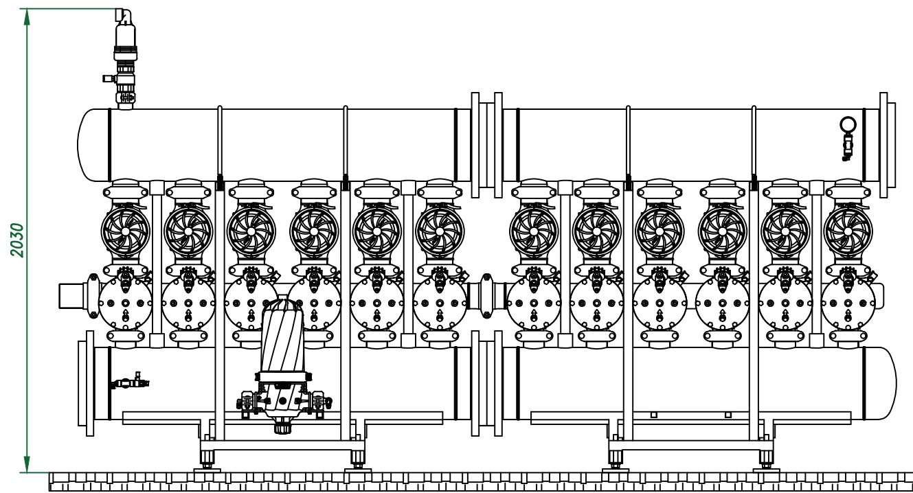
Вид спереди
